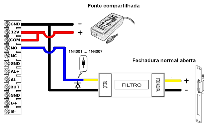
Ligação do filtro antirruídos (opcional)
