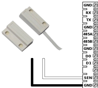
Ligação de sensor de porta aberta
