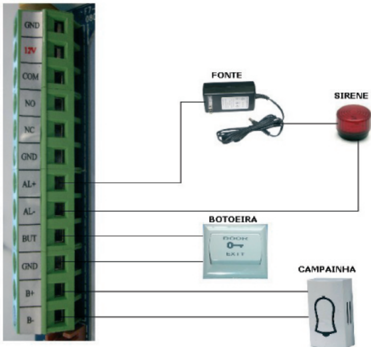
Desenho 2: Ligação de outros periféricos
